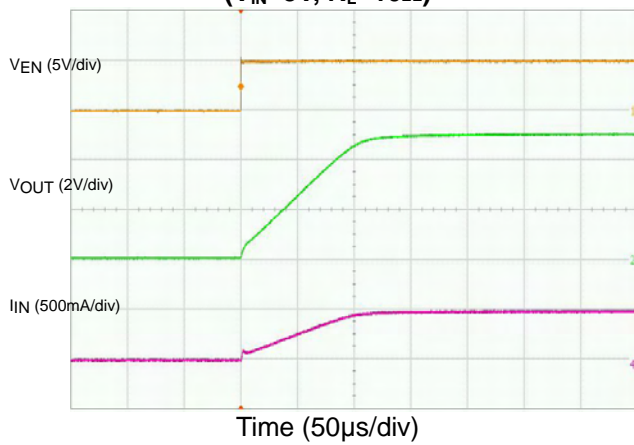
AP2281-3 Turn-On ( V_{IN}=5V , R_L=10\Omega )
