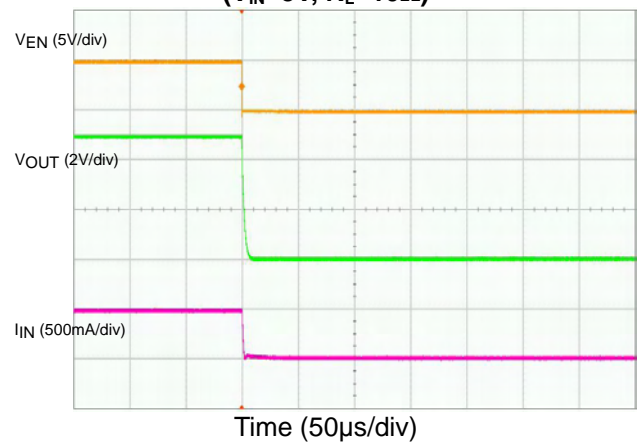
AP2281-3 Turn-Off ( V_{IN}=5V , R_L=10\Omega )
